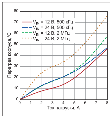
Рис. 9. Изменение температуры корпуса DC/DC-преобразователя LT8645S на примере оценочной платы DC2468A
