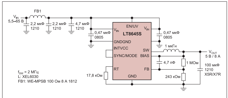
Рис. 4. Типовая схема включения LT8645S с расширением спектра рабочей частоты
