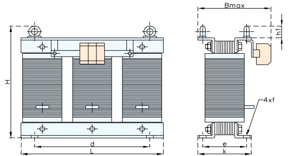
исполнение С для мощности 4,0 кВА и свыше
