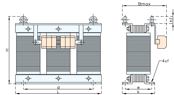
исполнение В для мощности 4,0 кВА и свыше
