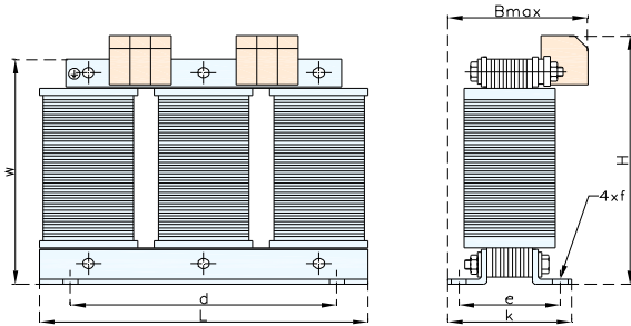
исполнение А для мощности до 4,0 кВА
