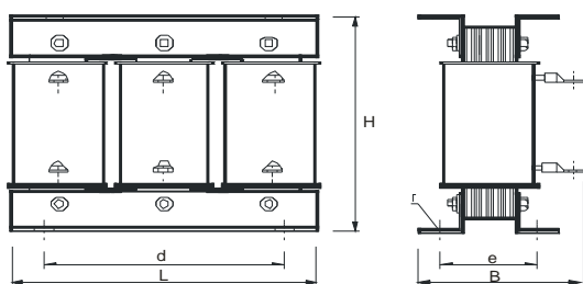
исполнение B
