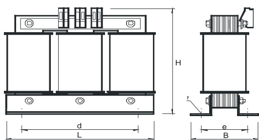
исполнение A
