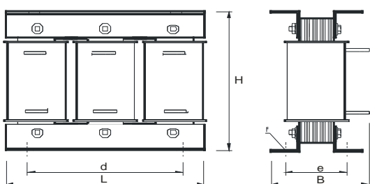
исполнение C
